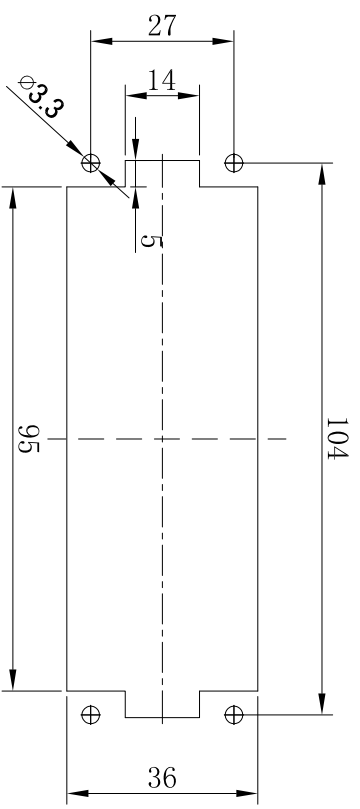
面板安装开孔图
