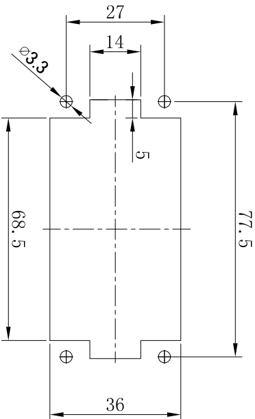
面板安装开孔图
