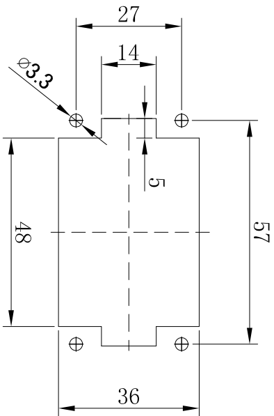
面板安装开孔图
