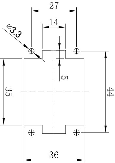
面板安装开孔图
